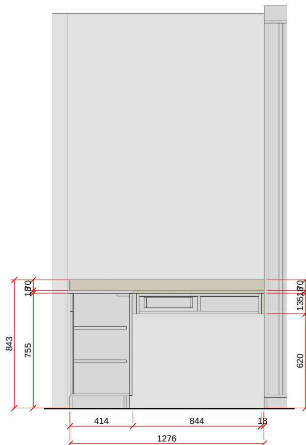
VISTA C - ESC. 1:25
