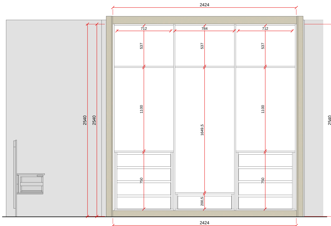
VISTA E - ESC. 1:25
