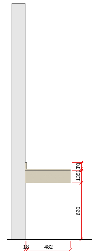
VISTA C - LATERAL - ESC. 1:25
