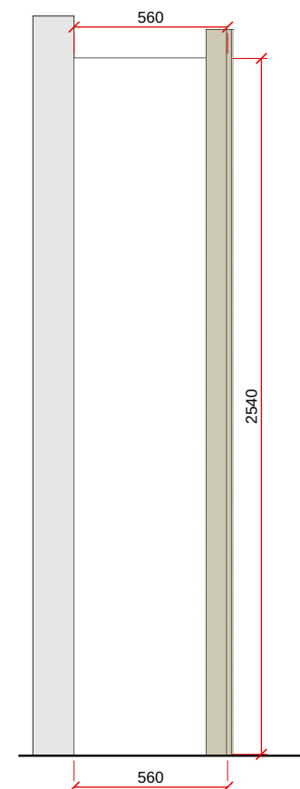
VISTA E - LATERAL - ESC. 1:25
